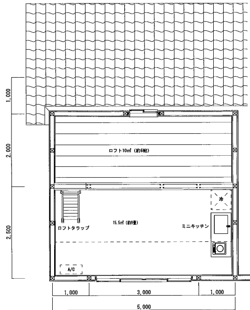
平面詳細図 2階ロフト部
