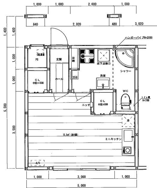
平面詳細図 1・2階共通
