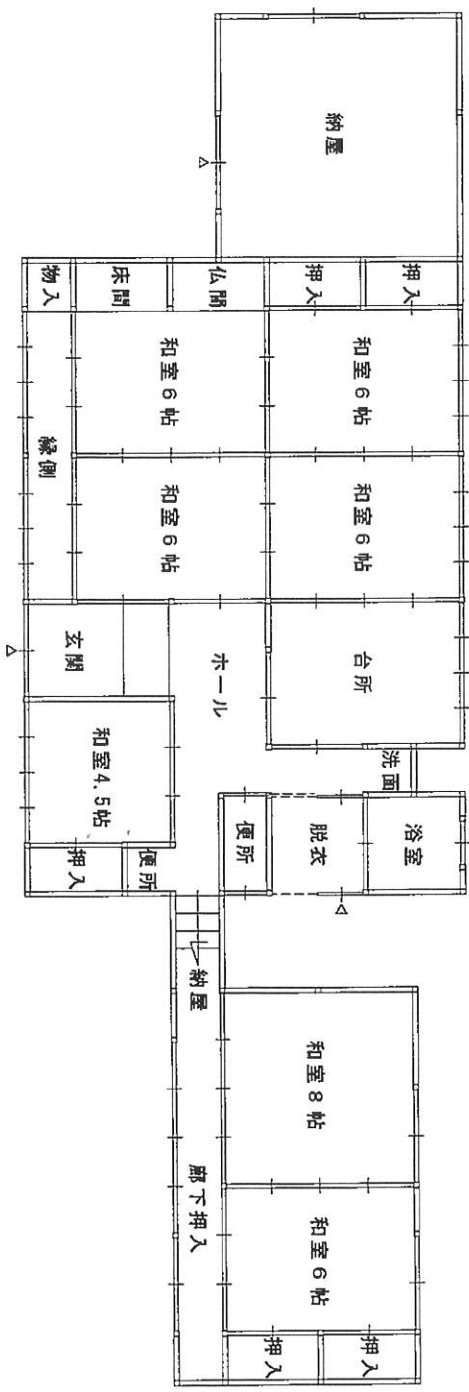
母屋 1階平面図
